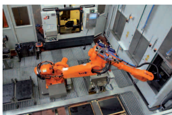
W1 Механическая обработка W1 mechanical machining
